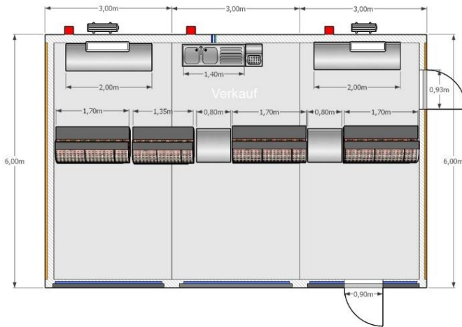
3er Verkaufsanlage 9x6m
