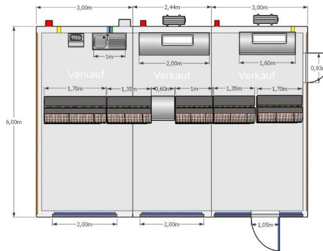
3er Verkaufsanlage 8,44x6m
