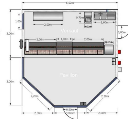
2er Verkaufsanlage 6x6m
